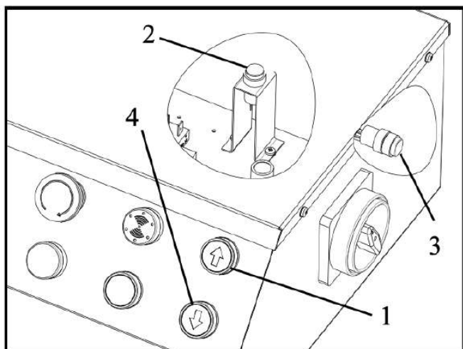
Fig. 6 - Luftning av hydrauliksystem och nivellering av billyften
