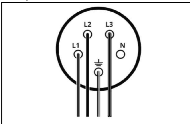
Fig. 5 - Tilslutning af 400V
