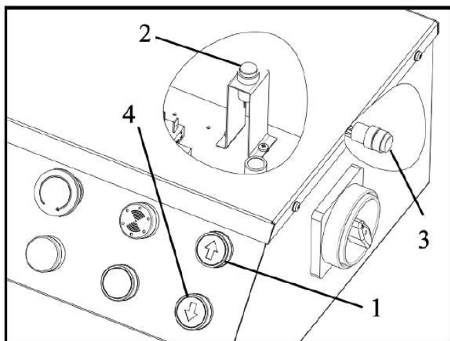
Fig. 6 - Udluftning af hydrauliksystem og nivellering af autoliften
