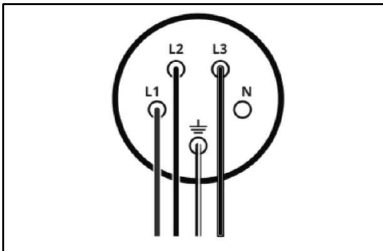
Fig. 5 - Anslutning av 400V
